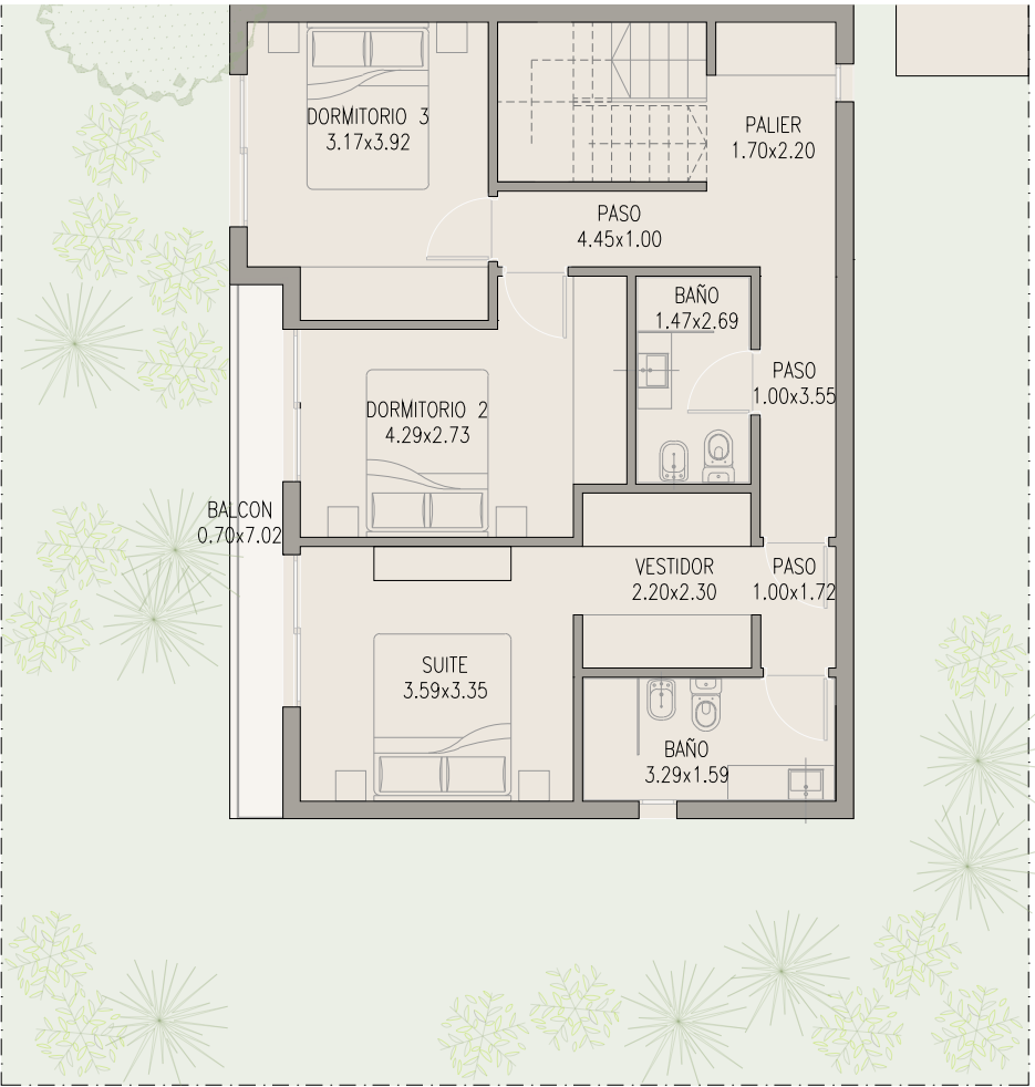
PLANTA ALTA
