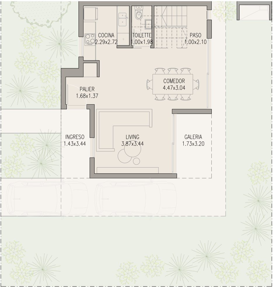
PLANTA BAJA
